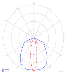
Lichtverteilung Linse Fluchtweg
