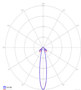
Lichtverteilung Linse Spot
