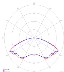
Lichtverteilung Linse Antipanic
